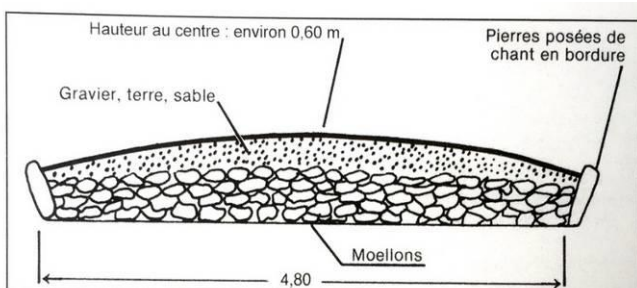
Fig. 145. La coupe de la voie romaine à Fontaulade, commune de Chadenac (d'après A. Mraile).
